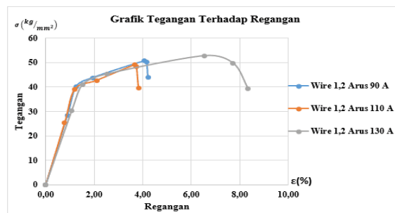
Gambar 23. Grafik Rata-Rata Tegangan dan Regangan Varisai Diameter Wire Ø1,2 Arus 90A, 110A, 130A
