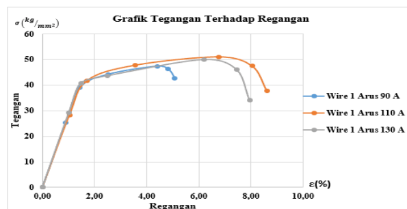
Gambar 21. Grafik Rata-Rata Tegangan dan Regangan Variasi Diameter Wire Ø1 Arus 90A, 110A, 130A
