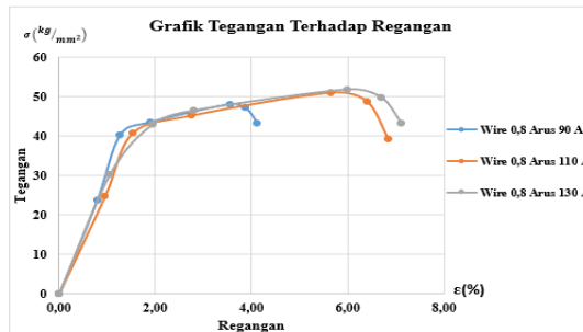
Gambar 19. Grafik Rata-Rata Tegangan dan Regangan Variasi Diameter Wire Ø 0,8 Arus 90A, 110A, 130A
