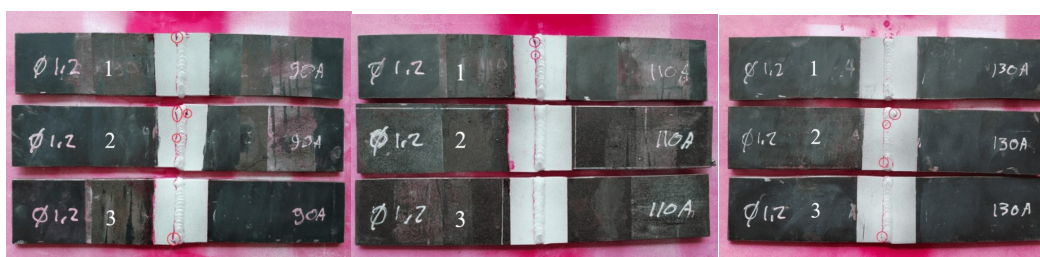
Gambar 15. Penetrasi Variasi Wire Ø1,2 Arus 90A, 110A, 130A
