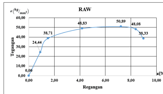
Gambar 17. Grafik Tegangan dan Regangan RAW
