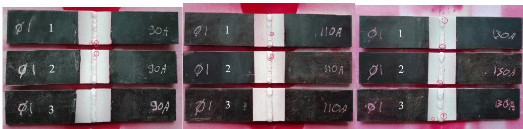
Gambar 14. Penetrasi Variasi Wire Ø1 Arus 90A, 110A, 130A
