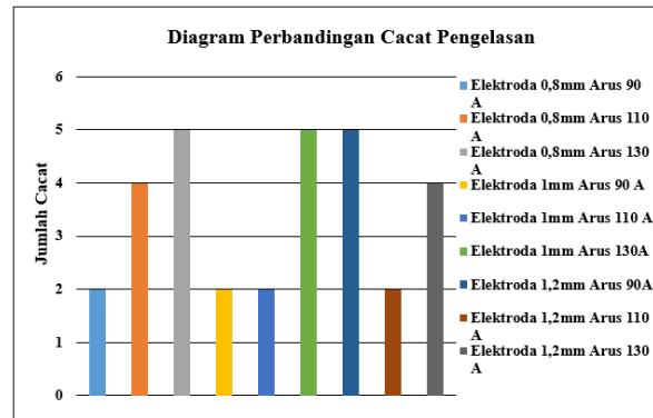
Gambar 16. Diagram Jumlah Cacat Setiap Variasi
