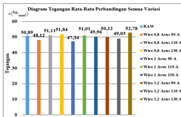
Gambar 24. Diagram Tegangan Rata-rata Semua Variasi
