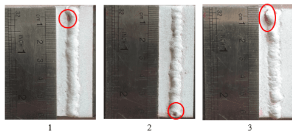
Gambar 113. Analisa Cacat Pengelasan Tungsten 1,6 mm Arus 120 A
