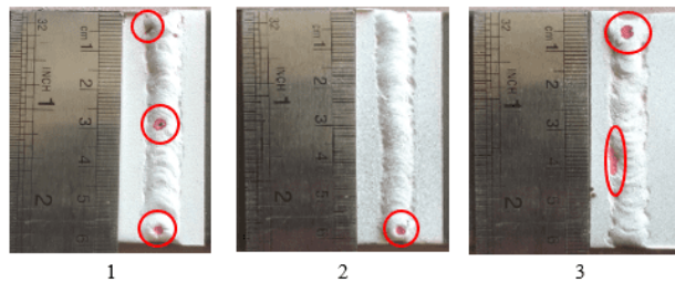
Gambar 116. Analisa Cacat Pengelasan Tungsten 2,4 mm Arus 100 A
