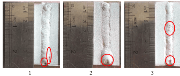
Gambar 115. Analisa Cacat Pengelasan Tungsten 2,4 mm Arus 100 A
