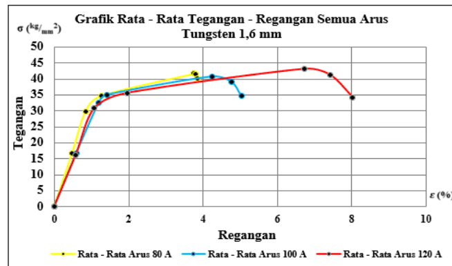
Gambar 21 Grafik Rata-Rata Tegangan – Regangan Tungsten 1,6 mm Arus 80 A, 100 A, 120 A
