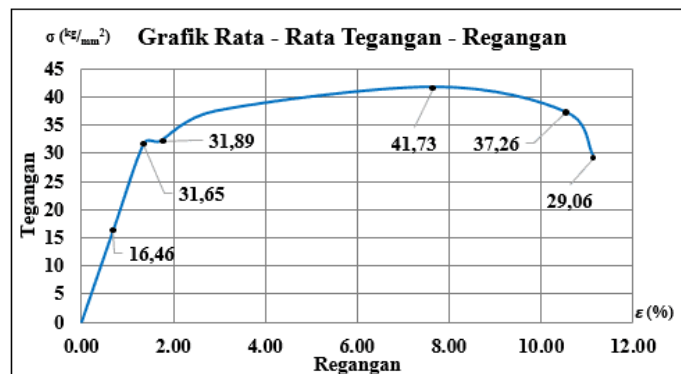
Gambar 20 Grafik Rata – Rata Tegangan – Regangan Raw Material
