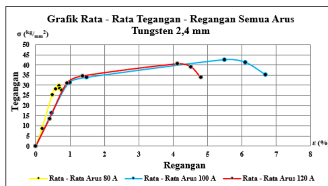
Gambar 22 Grafik Rata-Rata Tegangan – Regangan Tungsten 2,4 mm Arus 80 A, 100 A, 120 A
