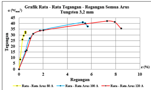
Gambar 23 Grafik Rata-Rata Tegangan – Regangan Tungsten 3,2 mm Arus 80 A, 100 A, 120 A
