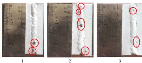
Gambar 117. Analisa Cacat Pengelasan Tungsten 3,2 mm Arus 80 A
