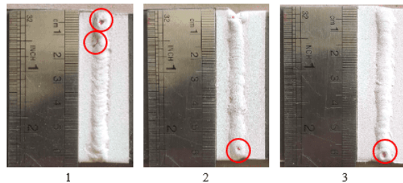
Gambar 112. Analisa Cacat Pengelasan Tungsten 1,6 mm Arus 100 A
