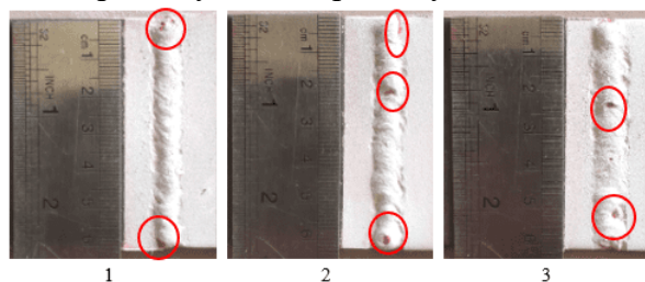
Gambar 114. Analisa Cacat Pengelasan Tungsten 2,4 mm Arus 80 A
