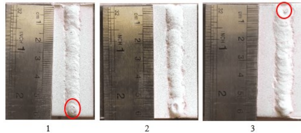
Gambar 119. Analisa Cacat Pengelasan Tungsten 3,2 mm Arus 120 A
