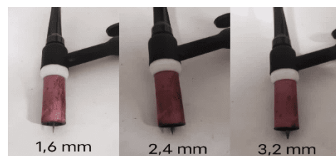
Gambar 2. Variasi Diameter Tungsten
