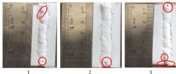
Gambar 118. Analisa Cacat Pengelasan Tungsten 3,2 mm Arus 100 A
