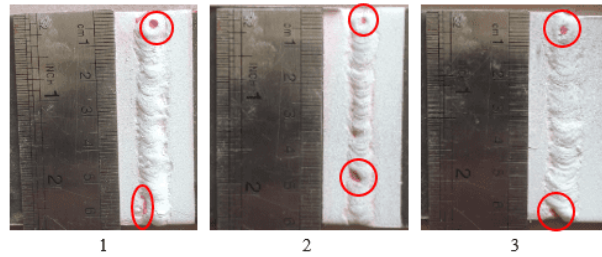
Gambar 111. Analisa Cacat Pengelasan Tungsten 1,6 mm Arus 80 A
