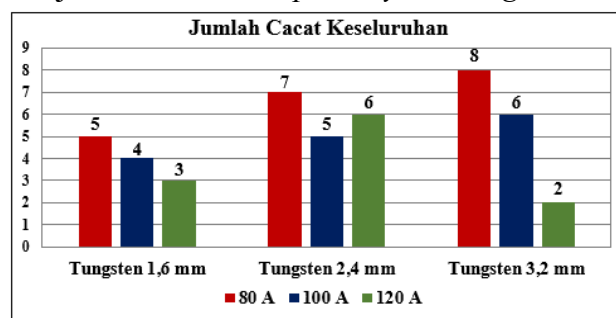
Gambar 20. Diagram Jumlah Cacat Keseluruhan
