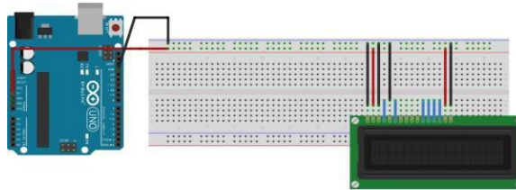
Gambar 8 Desain Arduino Uno Ke LCD
