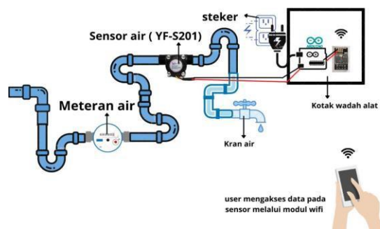
Gambar 7 Desain Keseluruhan Alat
