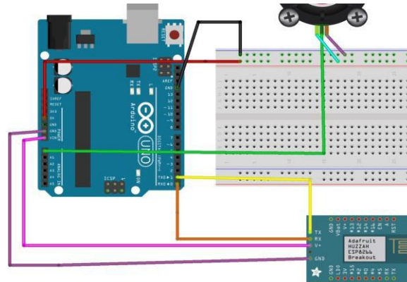
Gambar 9 Desain Arduino Uno ke ESP8266
