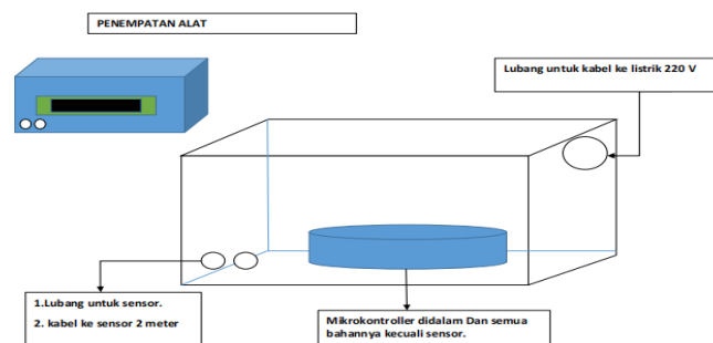
Gambar 12 Detail Penempatan Alat Di Box
