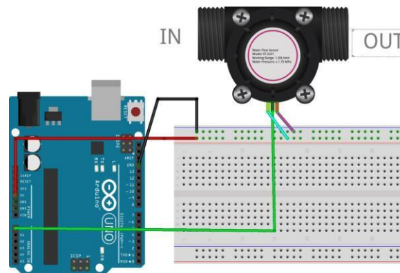
Gambar 10 Desain Rangkaian Sensor Aliran
