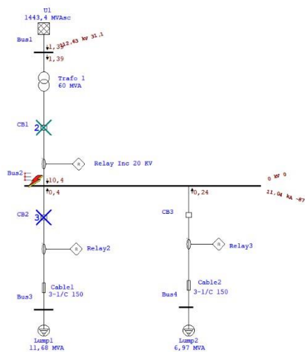
Gambar 3. Simulasi ETAP Pada Sisi Incoming
