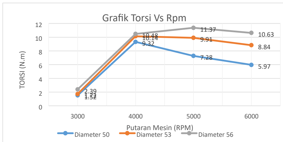
Gambar 8 Grafik analisis Torsi Vs Rpm
