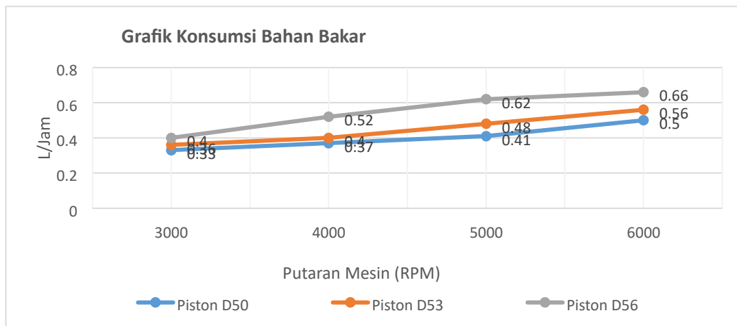
Gambar 10 Grafik konsumsi bahan bakar ( F_c ) Vs putaran mesin (RPM)
