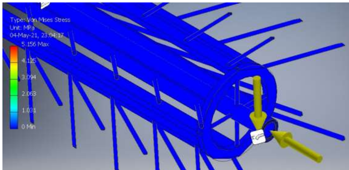
Gambar Hasil Ansys Silinder Perontok Pada Software
