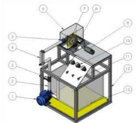
Gambar 2. Instalasi alat uji turbin pelton
