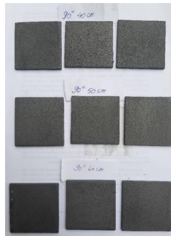
Gambar 9 Material uji setelah di proses sandblasting dengan variasi sudut 90 derajat dan jarak 40 cm, 50 cm, dan 60 cm
