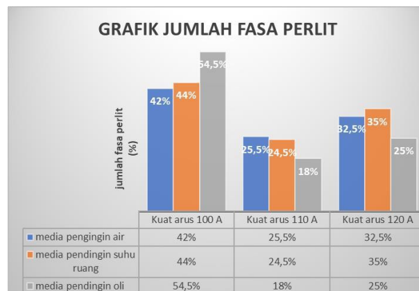
Gambar 15. Grafik Jumlah fasa perlit
