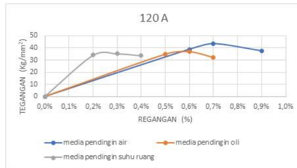
Gambar 9. grafik tegangan dan regangan dengan arus pengelasan 120 A
