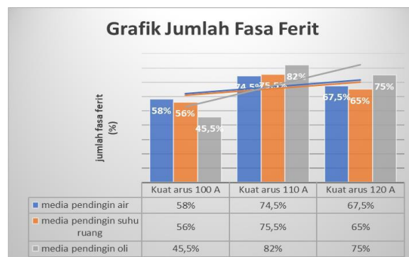
Gambar 13. trendline grafik jumlah fasa ferit
