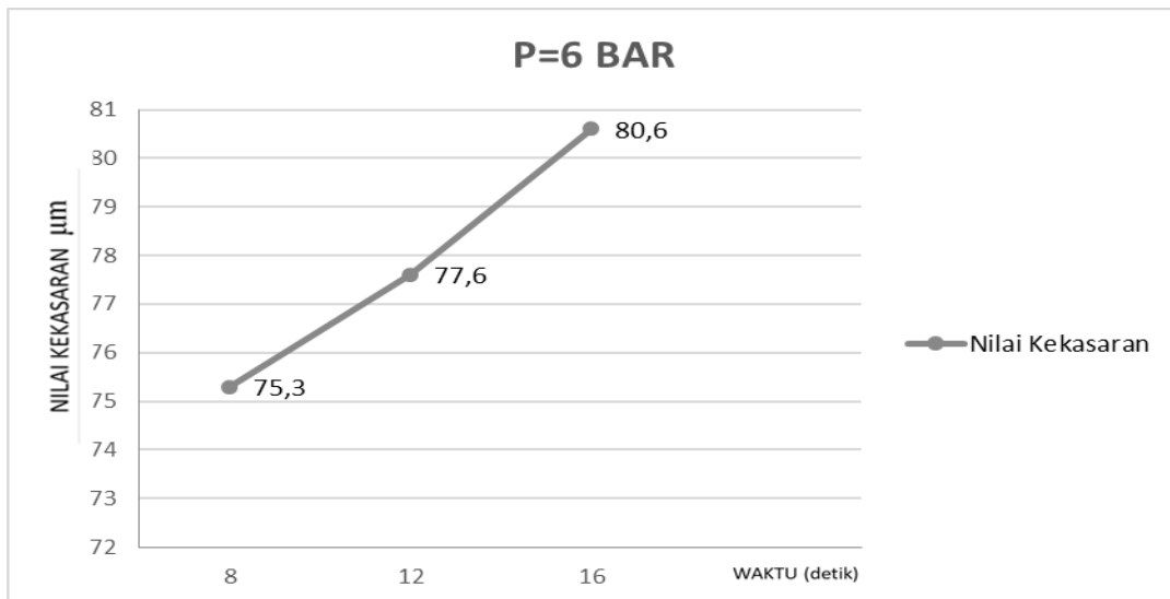
Gambar 15. Grafik tekanan 6 bar dengan waktu 8, 12 dan 16 detik.
