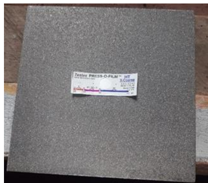
Gambar 12. Hasil proses sandblasting dengan tekanan 6 bar dan waktu 16 detik.
