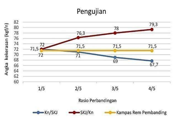
Gambar 12. Grafik Hubungan Hasil Pengujian Kekerasan
