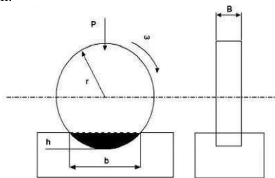
Gambar 8. Ilustrasi Pengujian Keausan Ogoshi
