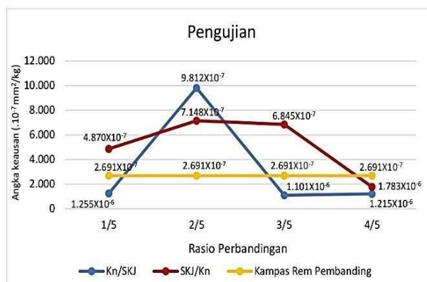
Gambar 15. Grafik Hubungan Hasil Pengujian Keausan
