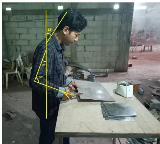
Gambar 18 Postur Kerja Operator Pemotong Manual
