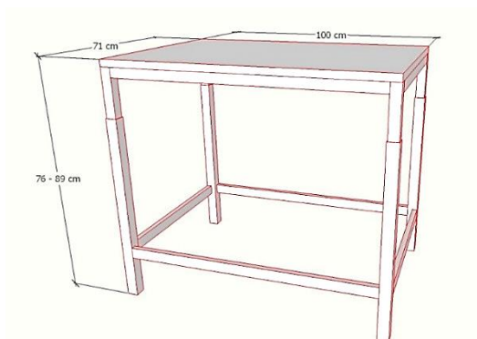
Gambar 13 Design Meja Kerja Pemotongan Manual
