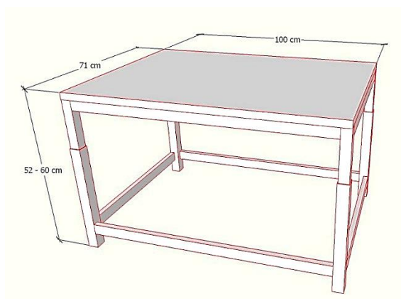
Gambar 12 Design Meja Kerja Mesin Bor
