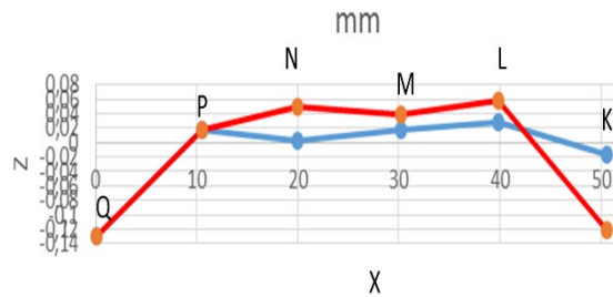
Gambar 8. Kedudukan titik-titik tampak belakang sebelum dan setelah T6 spesimen temperatur 400 0 dengan reduksi 5%
