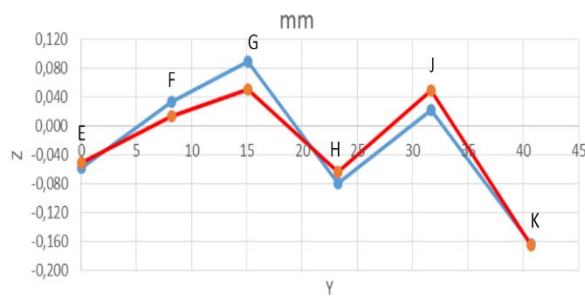
Gambar 5. Kedudukan titik-titik tampak kanan sebelum dan setelah T6 spesimen temperatur 400 0 dengan reduksi 5%
