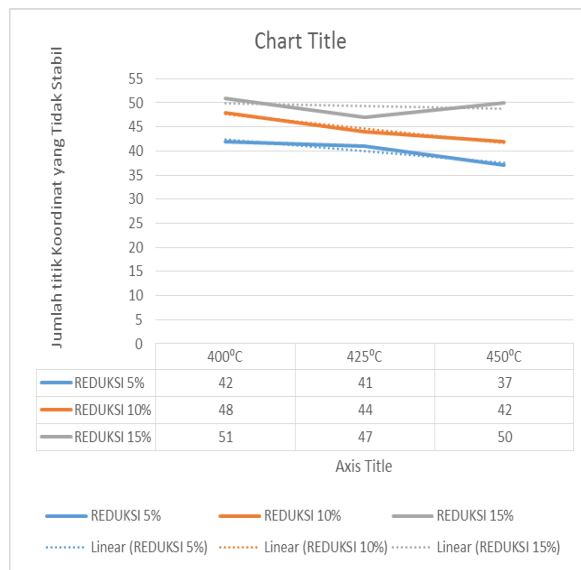
Gambar 9. Grafik pengaruh temperatur terhadap kestabilan titik-titik setiap spesimen
