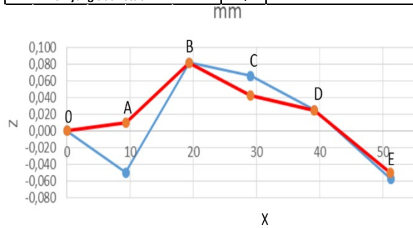
Gambar 4. Kedudukan titik-titik tampak depan sebelum dan setelah T6 spesimen temperatur 400 0 dengan reduksi 5%
