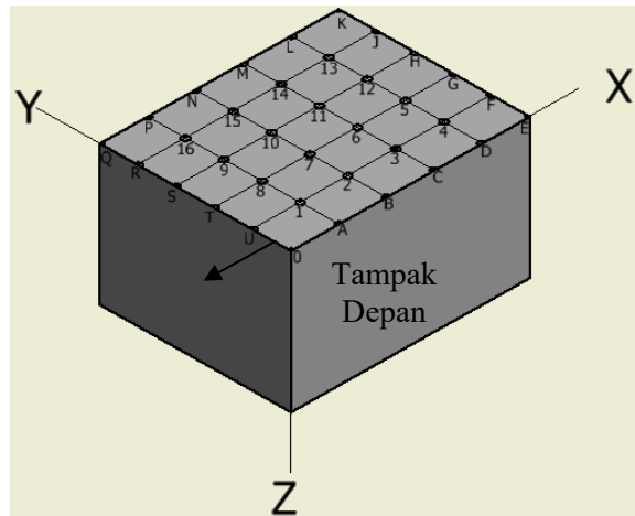
Gambar 2. Bentuk 3D spesimen dan lokasi koordinat yang diteliti
