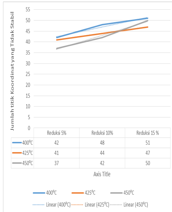
Gambar 10. Grafik pengaruh reduksi terhadap kestabilan titik-titik setiap spesimen
