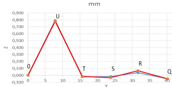
Gambar 6. Kedudukan titik-titik tampak samping kiri sebelum dan setelah T6 spesimen temperatur 400 o dengan reduksi 5%
